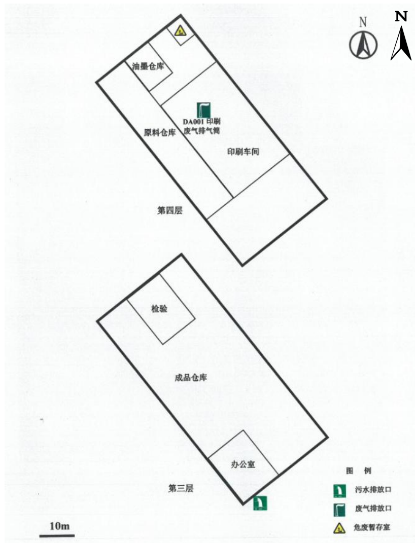
图 3-3 本项目平面布置图及生产车间平面布置图
